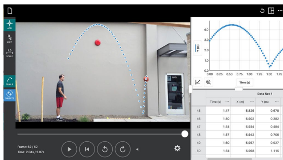
研究拋射運動
