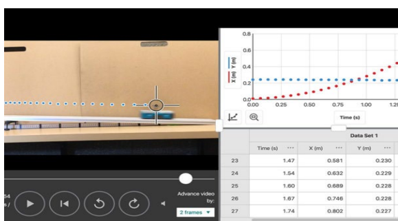
在實驗室中測量小車的加速度
